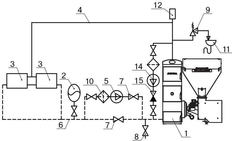
Рис.9 Схема закрытой системы отопления (рециркуляционная система с насосом)
